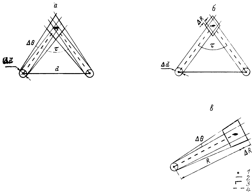
Рис. 6. Источники погрешности координат меченой рыбы для триангуляционного (а), дальномерного (б) и пеленгационно-дальномерного (в) способов пеленгации.
