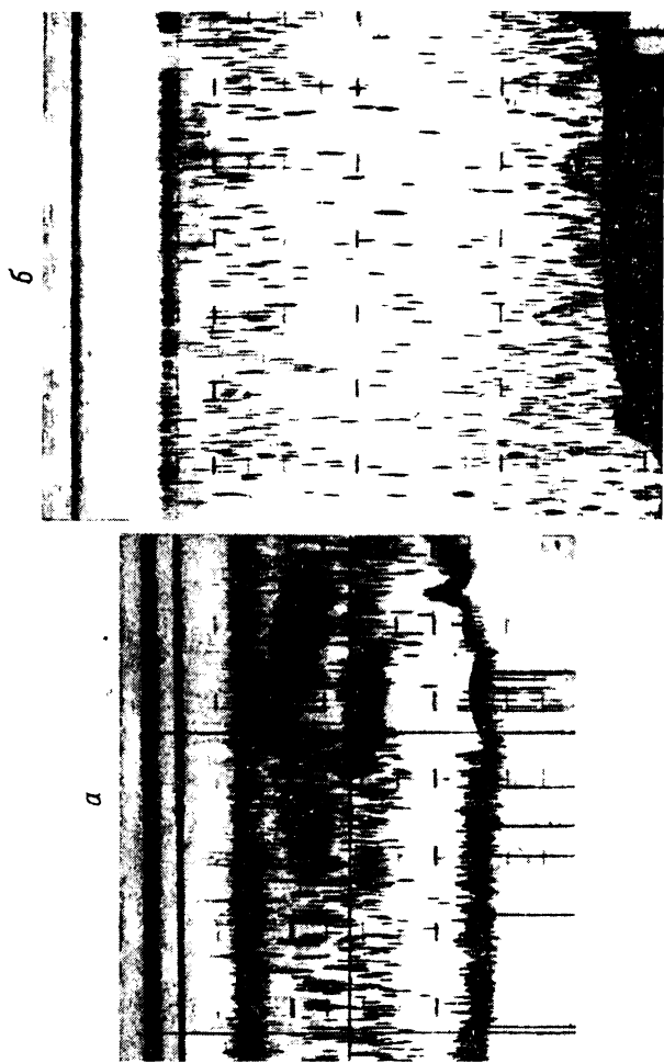
Рис. 21. Эхолозиль двустойного (а) и дисперсного (б) распределения рыб.
