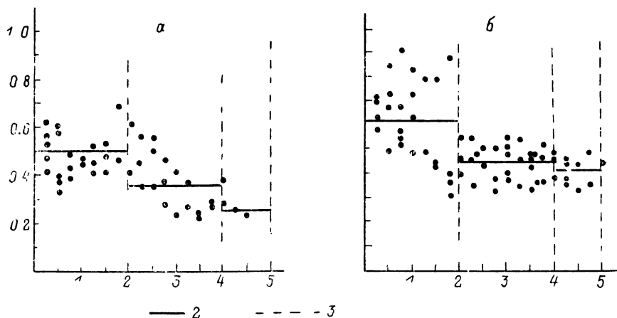
Рис. 105. Плотность рыб в пелагиали на пойменном плато водохранилища в районе затопленной реки (а) и в районе бывшего озера (б).
