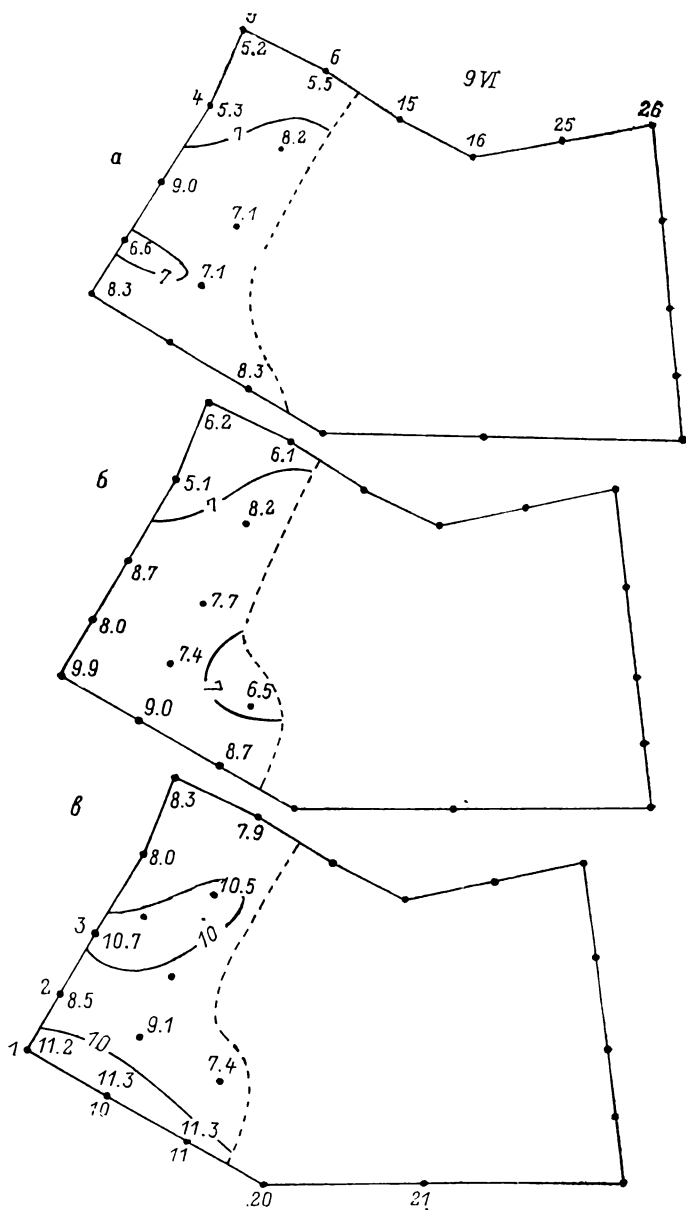
Рис. 14. Распределение концентраций хлорофилла (мкг/л) а — хлорофилл «а» чистый, б — хлорофилл «а» общий,
