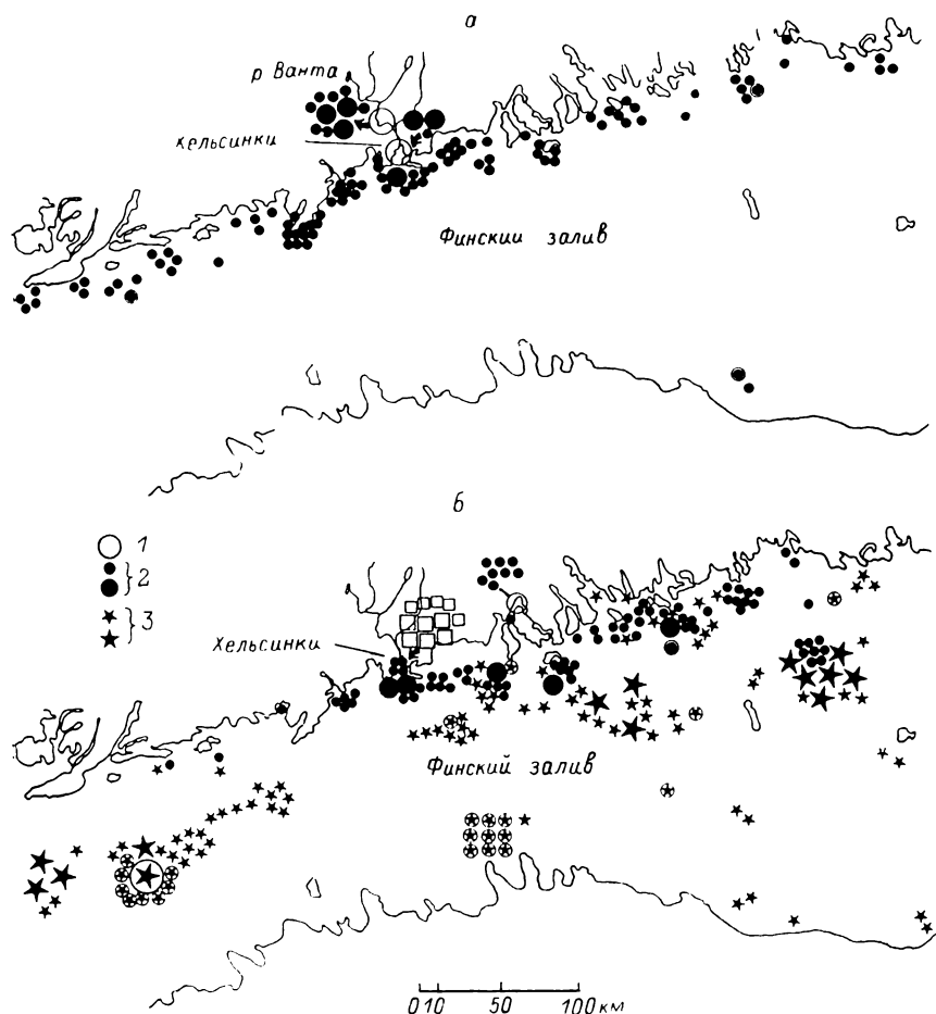
Рис. 40. Возврат меченых кумж (а) и лососей (б).
