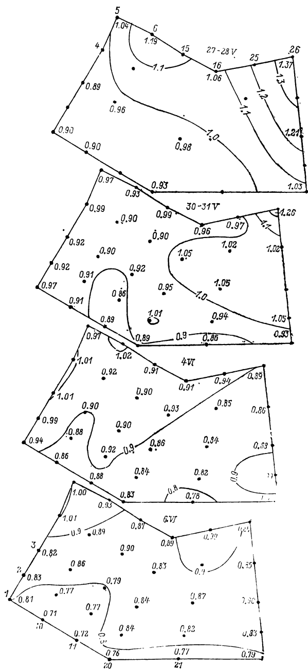
Рис. 19. Распределение пигментного отношения E_{480}/E_{664}
