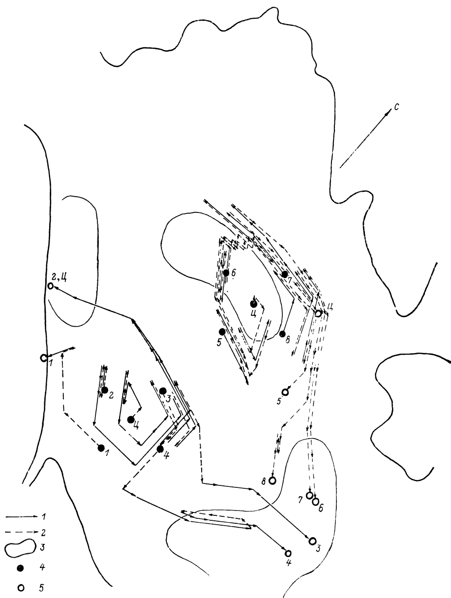
Рис. 52. Траектории перемещения единичных объемов воды при фактических ветрах в июне — августе 1987 г. в западной части Рыбинского водохранилища. 1 — циклонический перенос; 2 — антициклонический перенос; 3 — зоны наименьших скоростей переноса; 4 — начальное положение объемов воды; 5 — конечное положение объемов воды.
