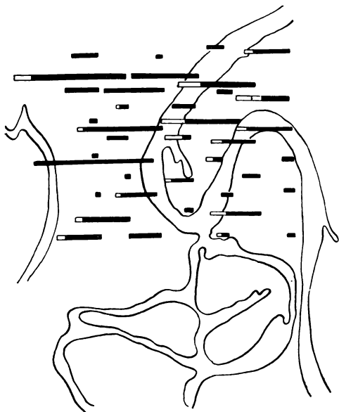
Рис. 29. Распределение биомассы бентоса на микрополигоне.
