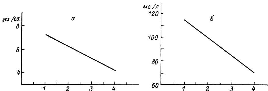
Рис. 87. Линия регрессии зависимости интенсивности питания окуня (а) и леща (б) от плотности посадки растительности в аквариуме.
