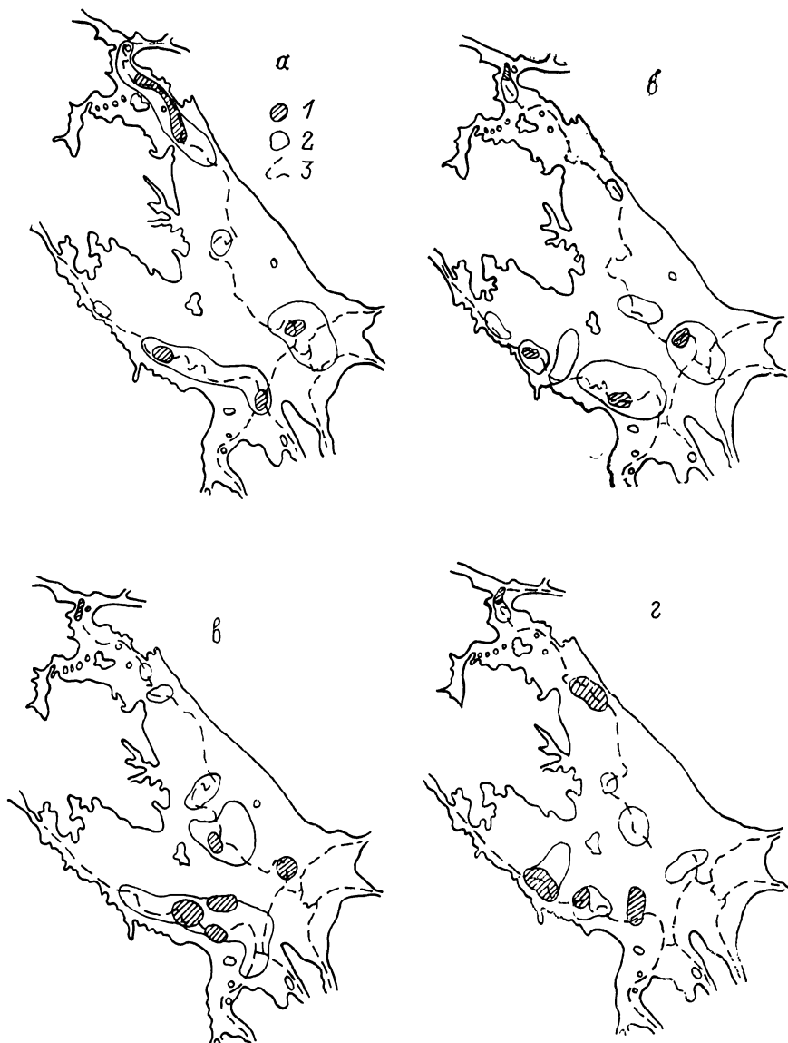
Рис. 23. Распределение наиболее плотных скоплений рыб в придонном слое а — август 1978 г., б — август 1979 г., в — август 1982 г., г — август 1984 г., остальные обозначения те же, что и на рис. 22.
