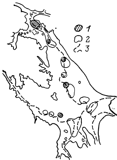
Рис. 24. Распределение наиболее плотных скоплений рыб в придонном горизонте в июле 1987 г.
