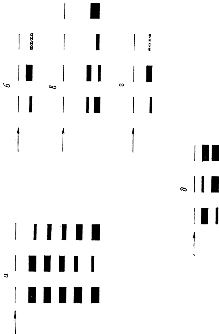
Рис. 91. Основные регуляторные типы изоферментов карповых рыб. а — ЛДГ; б — β-ЭСТ-1; в — β-ЭСТ-2; г — β-ЭСТ-3; д — По (по локусам МЭ регуляторные эффекты не обнаружены).
