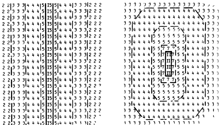
Рис. 104. Результаты математического моделирования распределения рыб на полигоне.
