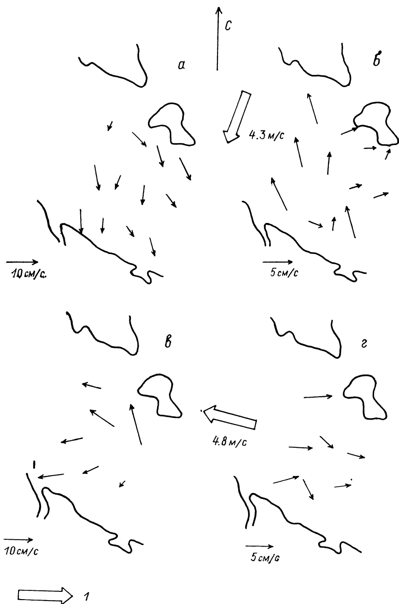
Рис. 10. Распределение векторов течений на полигоне 19 VI 84 в слое 0—2 м ( a ), глубже 4 м ( б ) и 16 VI 85 в слое 0—2 м ( в ), глубже 4 м ( г ).
