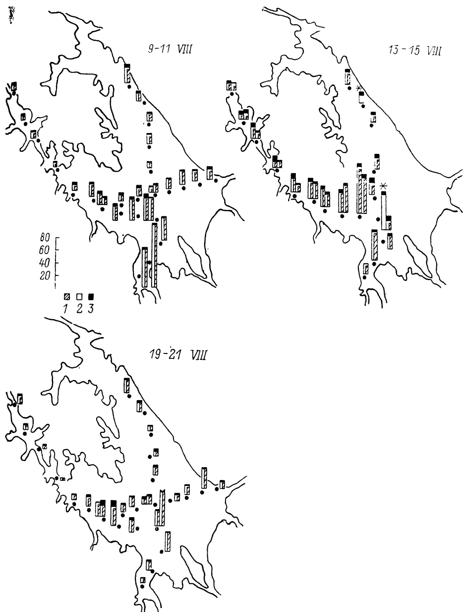
Рис. 13. Распределение хлорофилла ( \mu\text{кг/л} ) по акватории водохранилища летом 1986 г.
