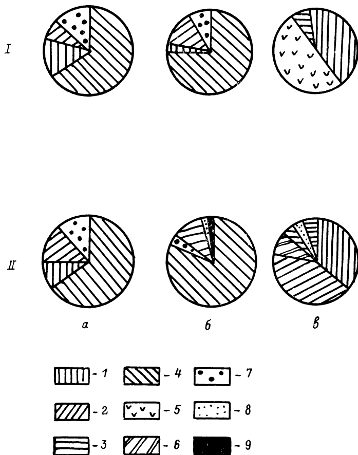
Рис. 62. Состав бентоса (а) и спектры питания леща (б) и ерша (а) на разных биотопах Рыбинского водохранилища в июне 1986 г. % по массе.
