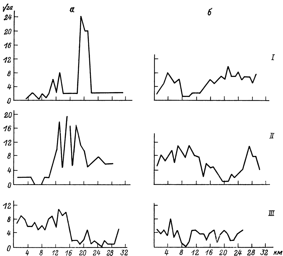
Рис. 31. Изменение плотности рыб (м) на 2 смежных (а, б) трансектах микрополигона по трем горизонтам воды.
