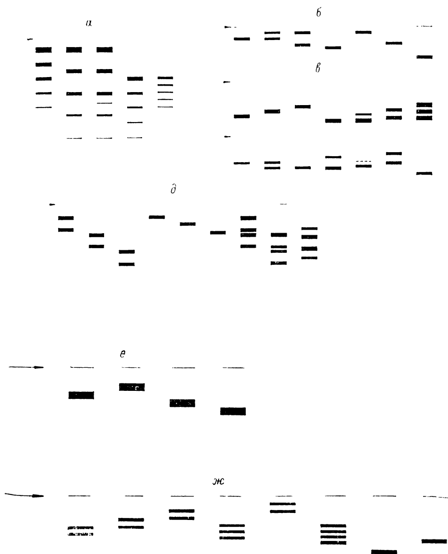
Рис. 90. Основные структурные типы изоферментов карповых рыб. \alpha — ЛДГ; \sigma - \beta ЭСТ-1, \alpha - \beta — ЭСТ-2, \epsilon - \beta — ЭСТ-3; \partial — По; \epsilon — МЭ-1, МЭ-2.
