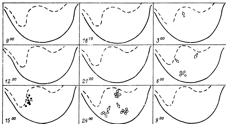
Рис. 73. Суточные перемещения плотвы и окуня в зоне зарослей в первых декадах июня (а) и июля (б), в третьей декаде июля (в).
